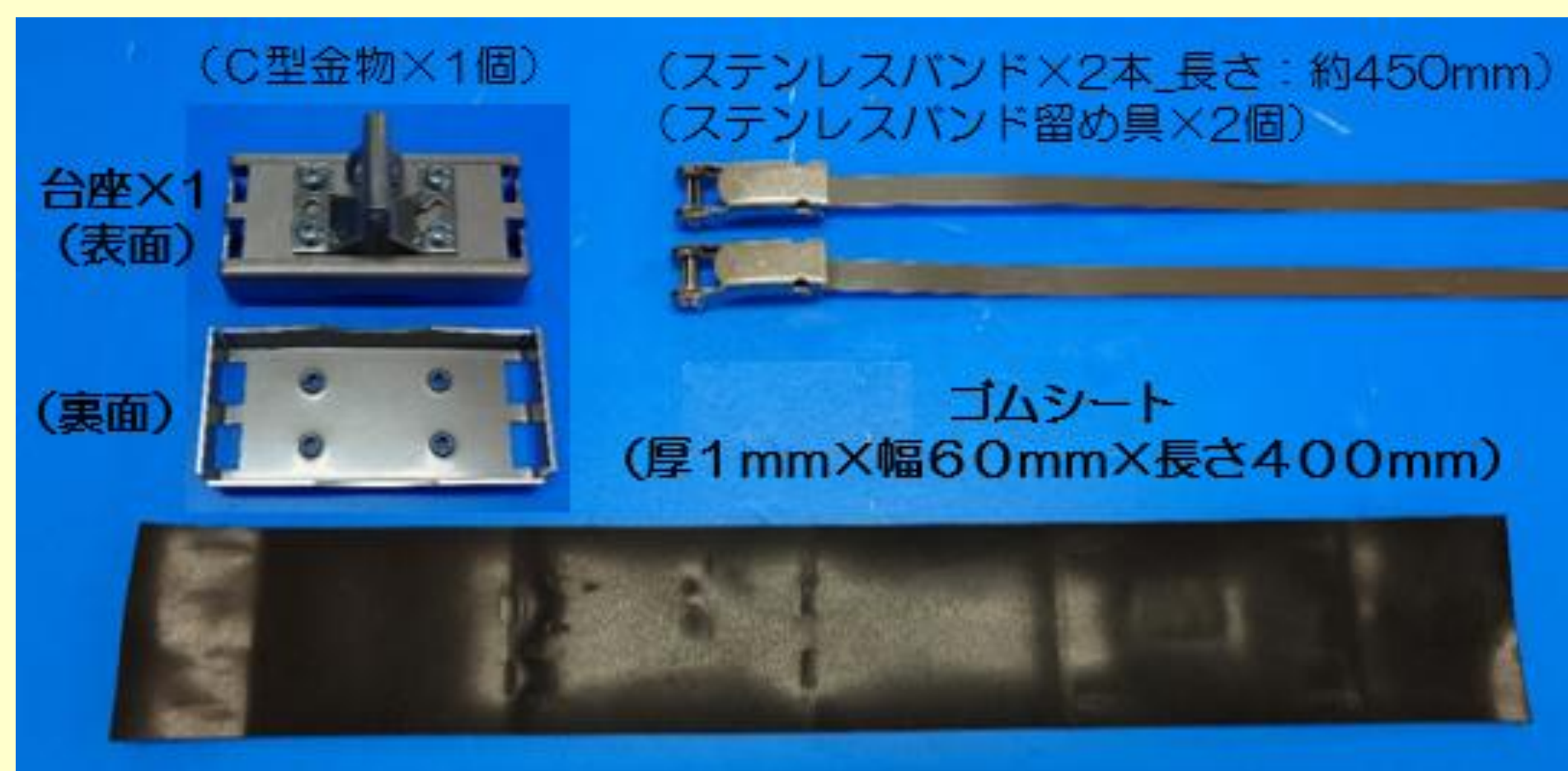
ベランダ用C型金物固定台座
