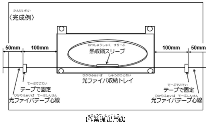
図2 光ファイバー作業試験課題
